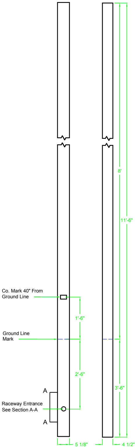
Pole Details SCALE: 1/2" = 1'
