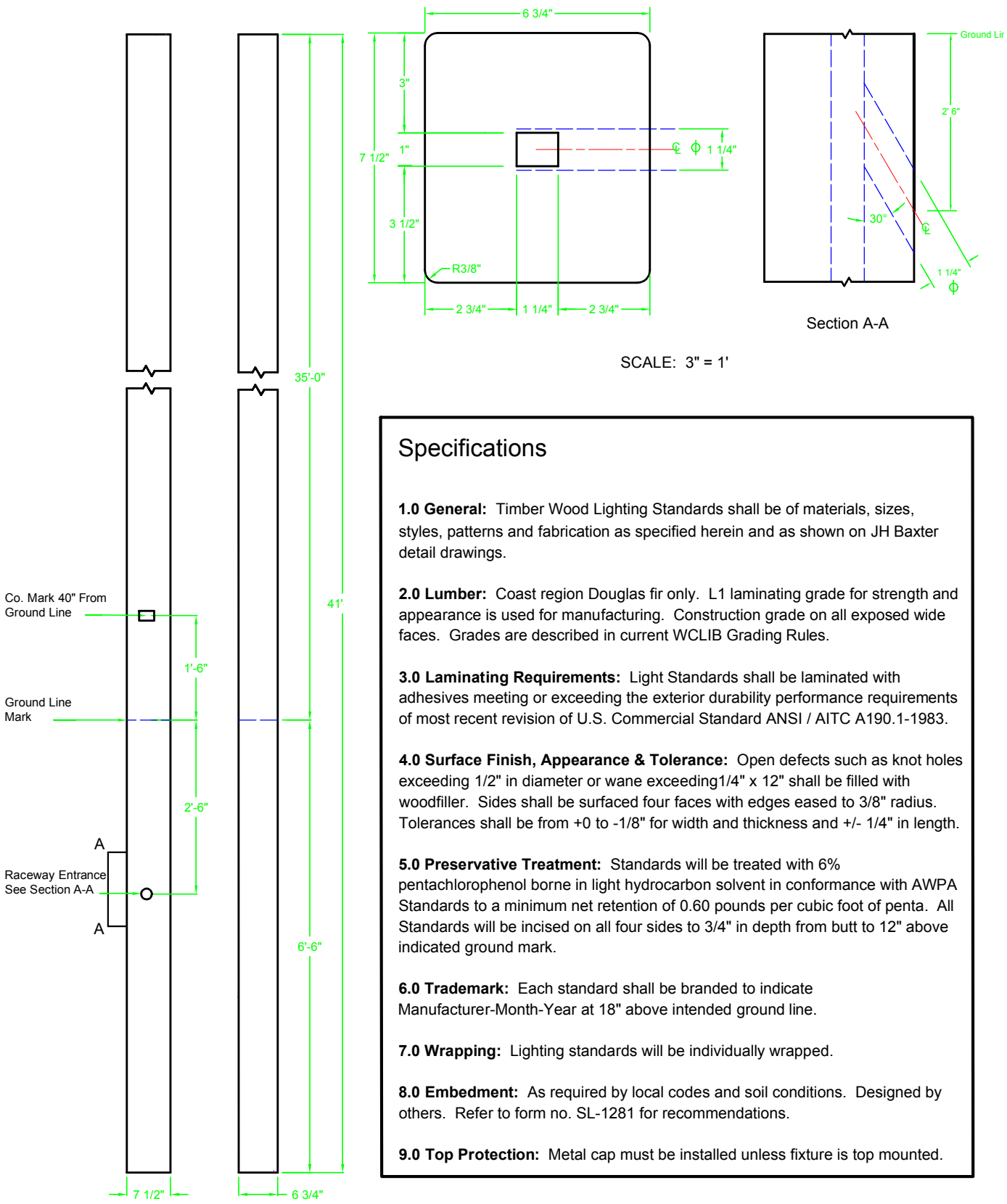
Pole Details SCALE: 1/2" = 1'
