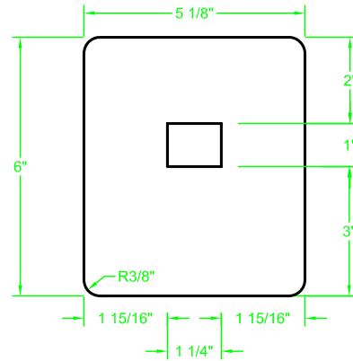
SCALE: 3" = 1'
