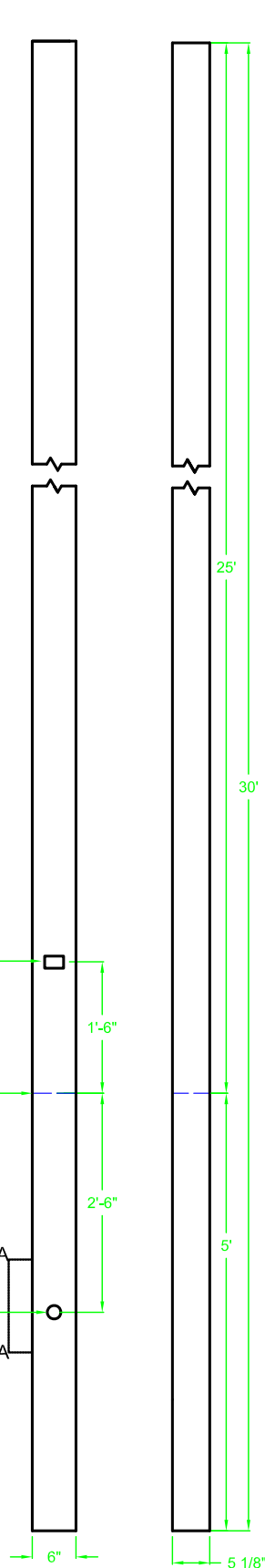
Pole Details SCALE: 1/2" = 1'
