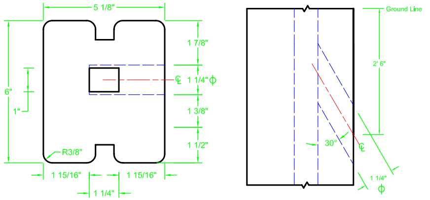
SCALE: 3" = 1'
