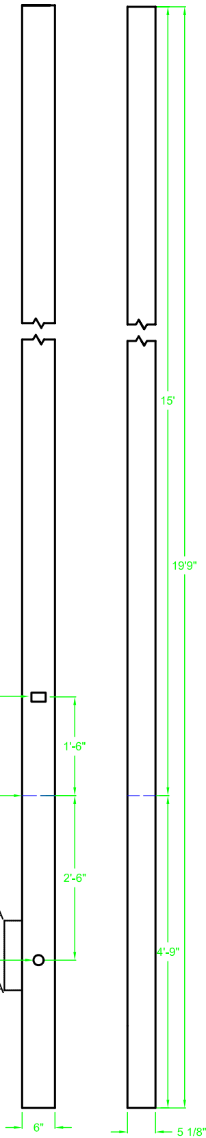
Pole Details SCALE: 1/2" = 1'
